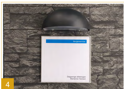
4 Alugraf Ultra - B: 210mm x H: 200mm
